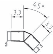
Profilo di congiunzione / Junction profile
